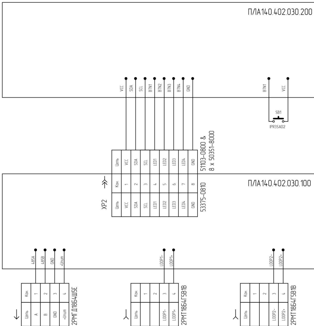
Приложение 2. Схема электрическая подключения Приемопередатчика 2,4 ГГц(А)
