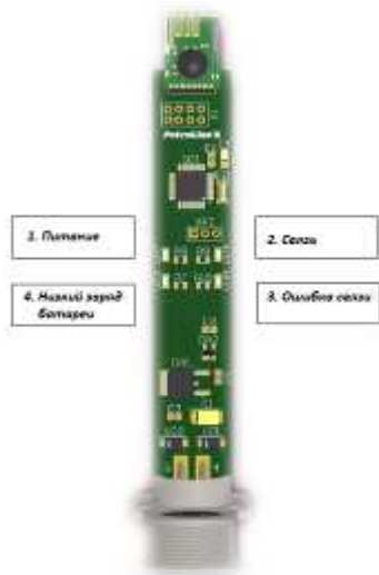
Рисунок 9. Приёмопередатчик ДКМ-140(Р)
