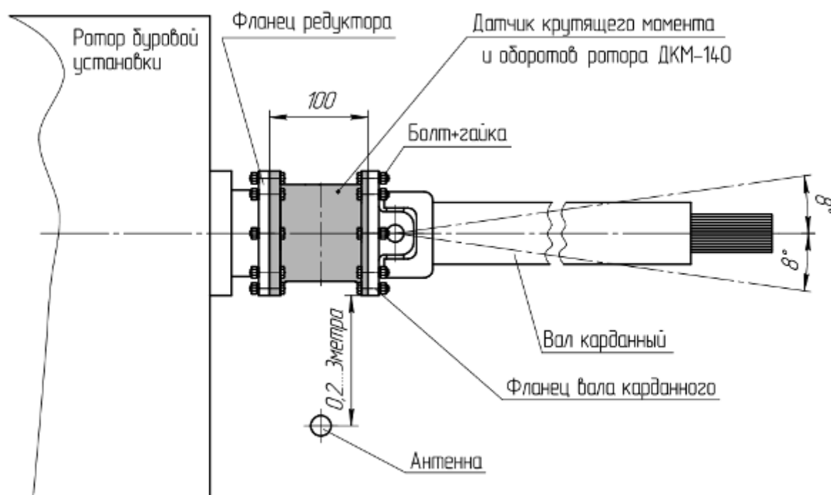
Рисунок 7. Схема монтажа ДКМ-140(Р)
