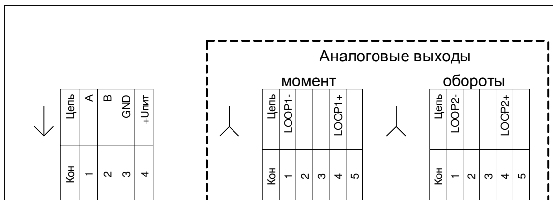
Рисунок 11. Схема электрическая подключения
